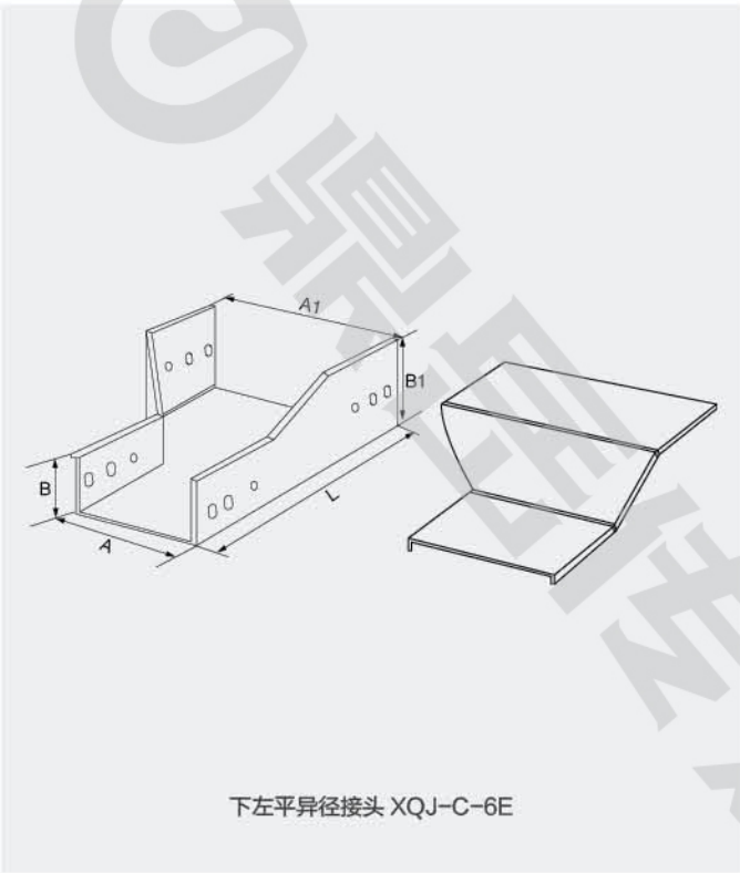
下左平异径接头
