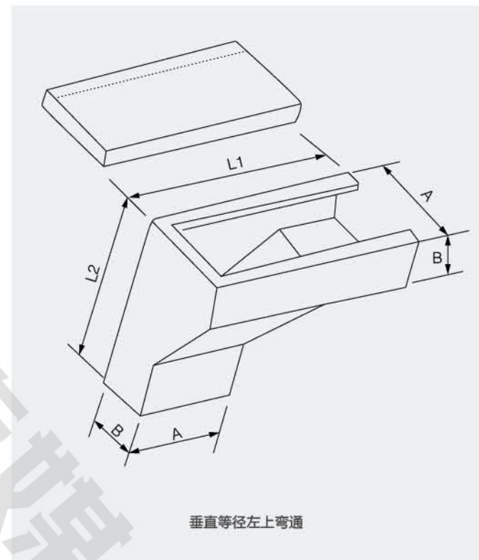
垂直等径左上弯通
