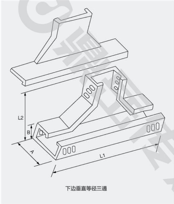
下边垂直等径三通
