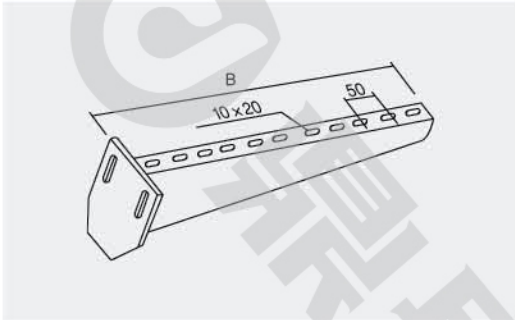
托臂 XQJ-TB-02
