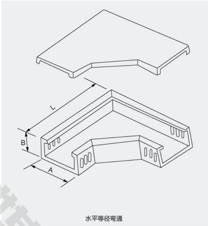
水平等径弯通
