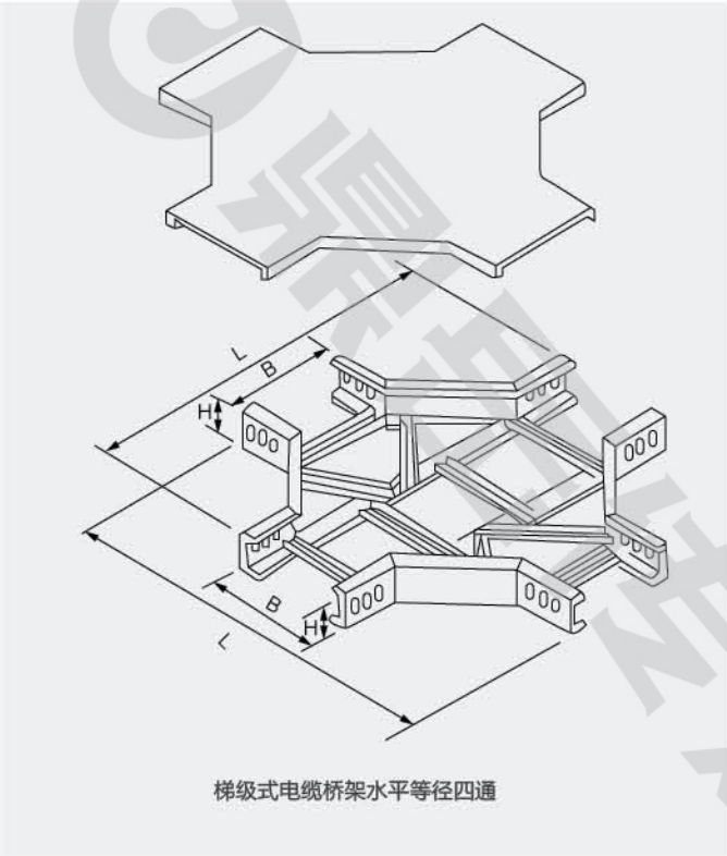
梯级式电缆桥架水平等径四通
