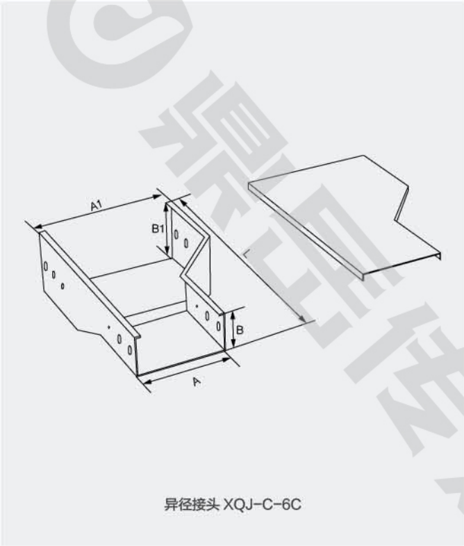
异径接头
