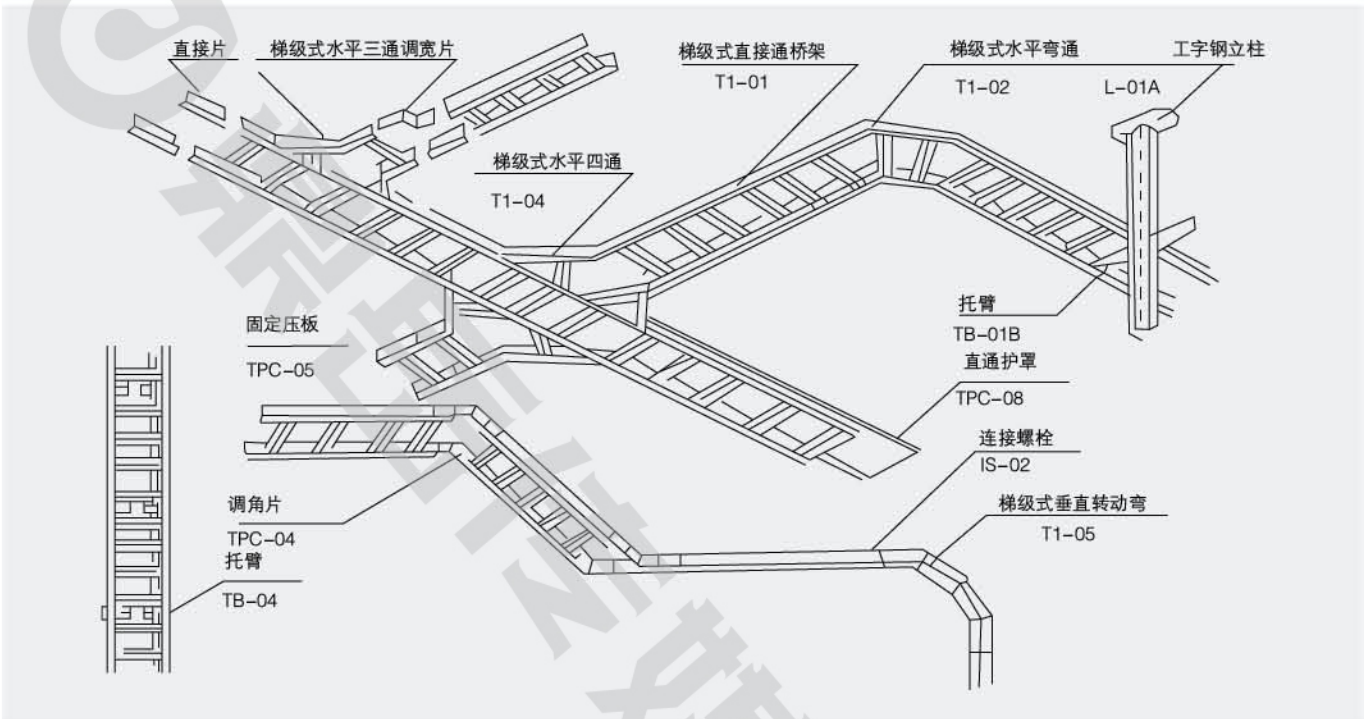
梯级式桥架空间布置示意图
