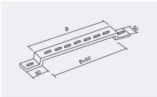
托臂 XQJ-TB-04
