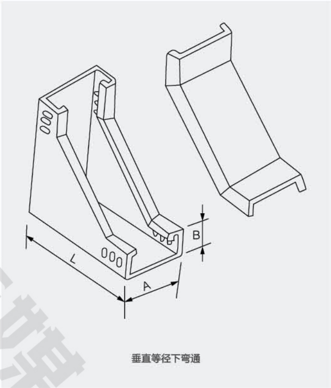
垂直等径下弯通
