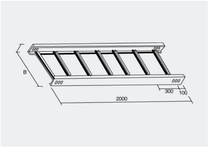
梯级式直通桥架 XQJ-T1-01
