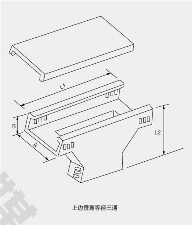
上边垂直等径三通
