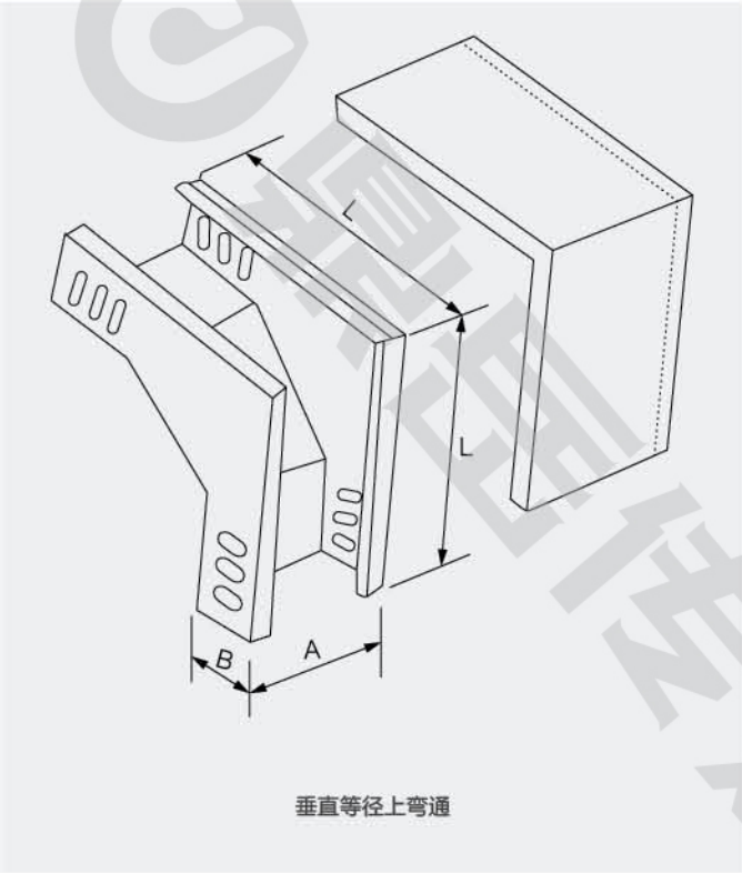
垂直等径上弯通
