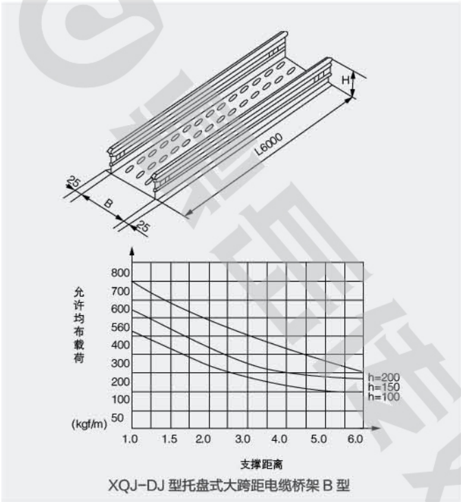
XQJ-DJ 型托盘式大跨距电缆桥架 B 型
