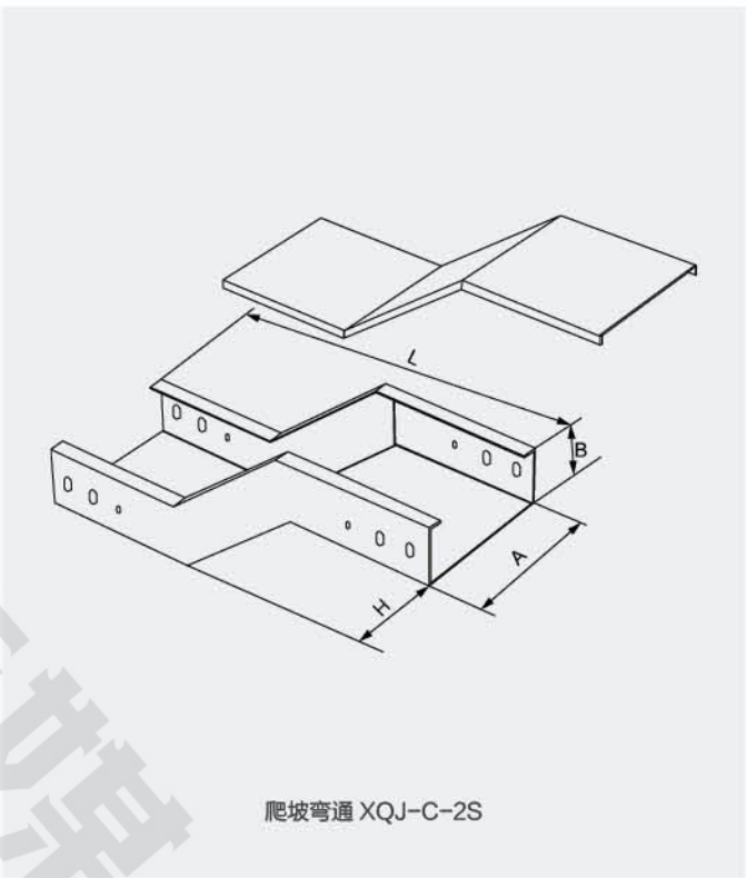
爬坡弯通
