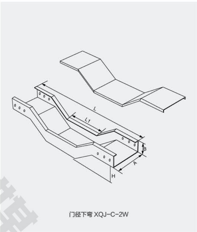
门径下弯
