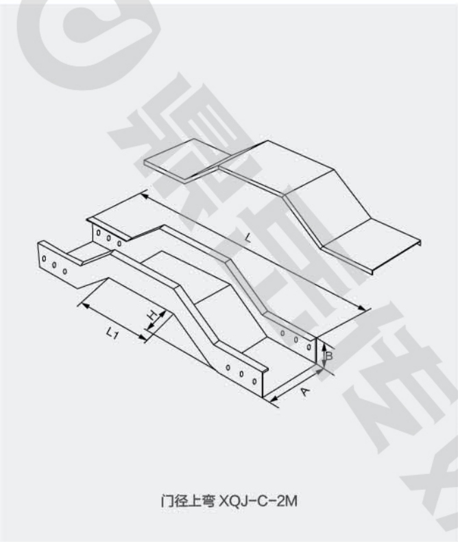
门径上弯
