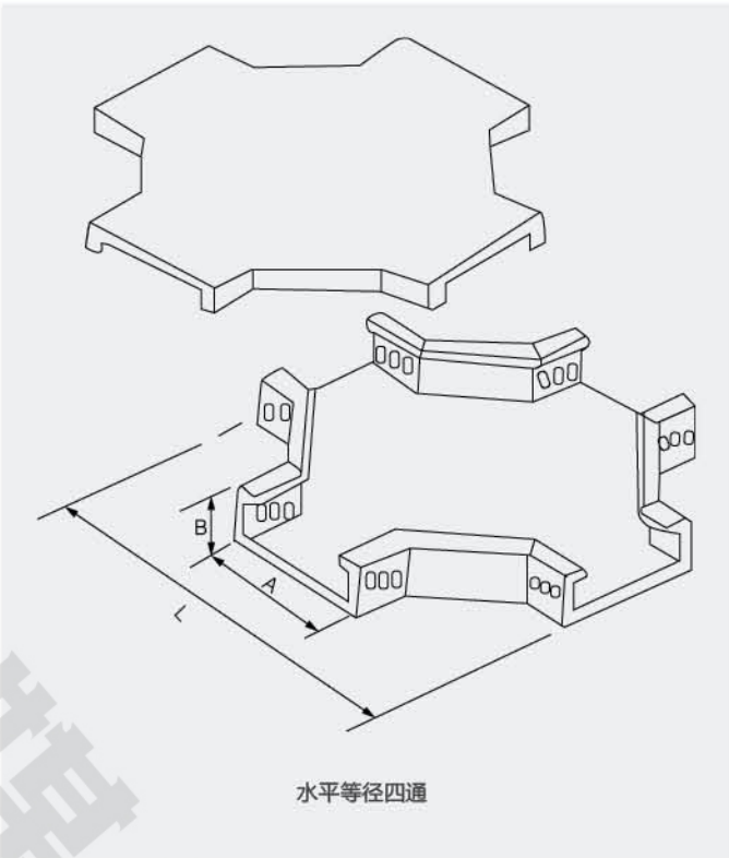
水平等径四通
