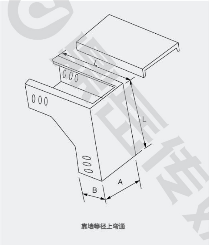
靠墙等径上弯通
