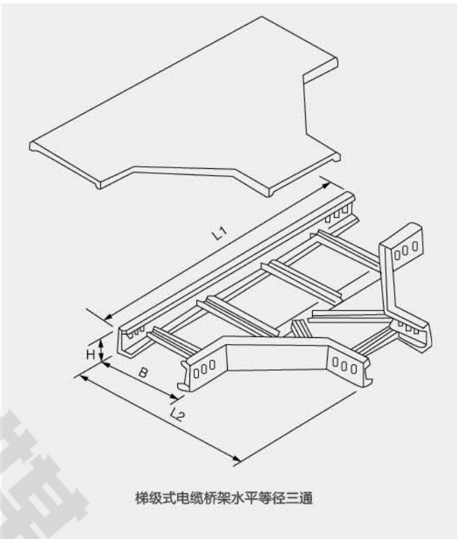
梯级式电缆桥架水平等径三通
