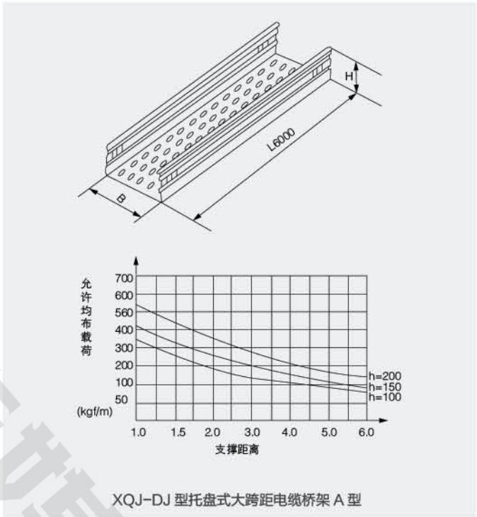
XQJ-DJ 型托盘式大跨距电缆桥架 A 型
