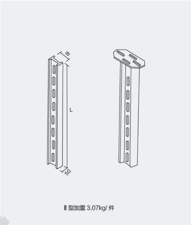
工字钢立柱 XQJ-H-01A
