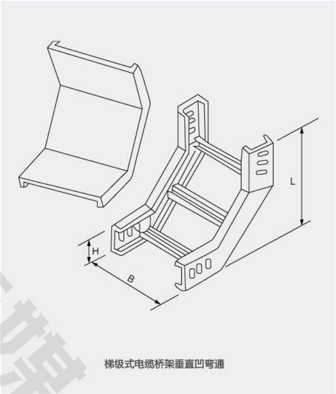
梯级式电缆桥架垂直凹弯通
