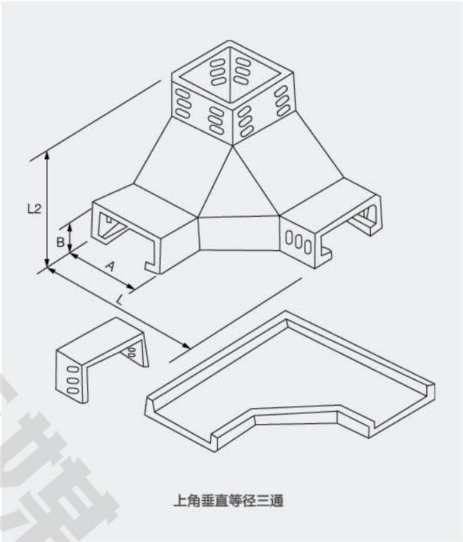
上角垂直等径三通
