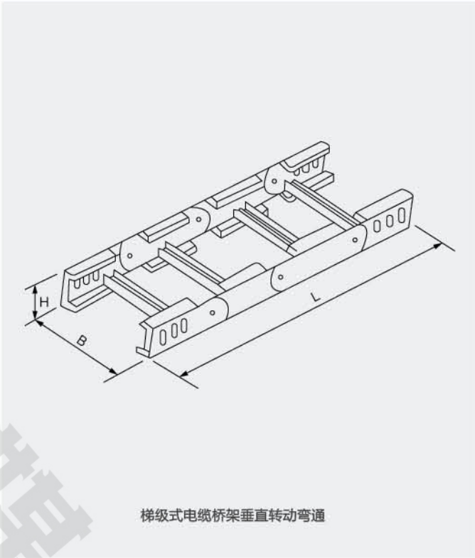
梯级式电缆桥架垂直转动弯通
