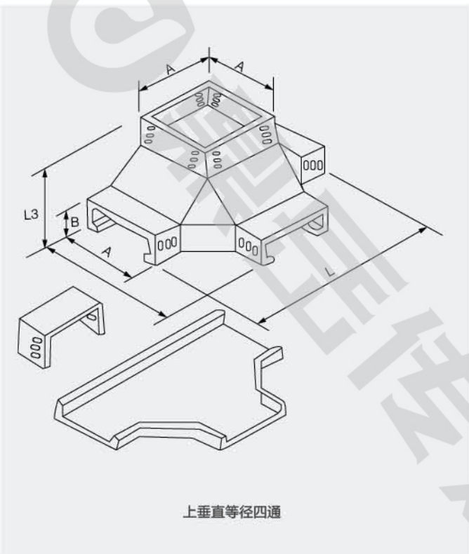
上垂直等径四通
