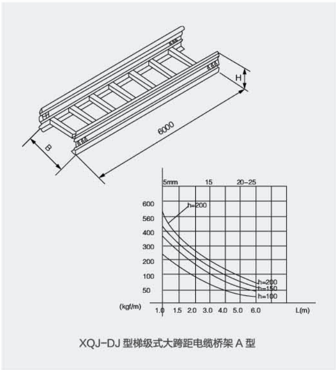
XQJ-DJ 型梯级式大跨距电缆桥架 A 型
