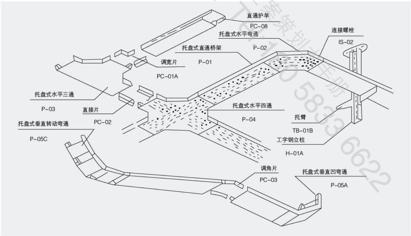
托盘式桥架空间布置示意图
