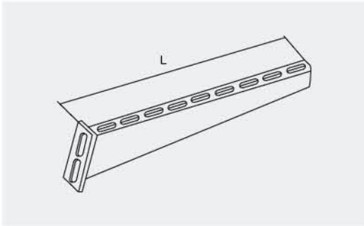
托臂 XQJ-TB-03
