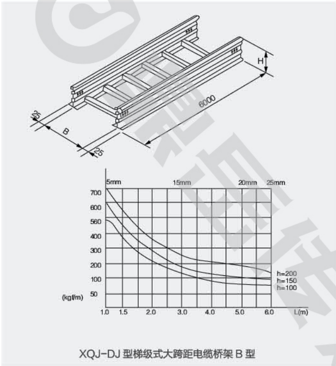
XQJ-DJ 型梯级式大跨距电缆桥架 B 型
