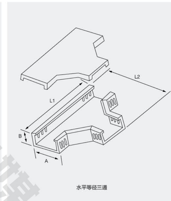
水平等径三通
