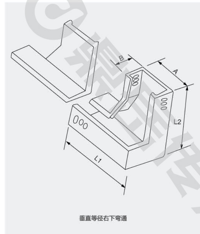
垂直等径右下弯通
