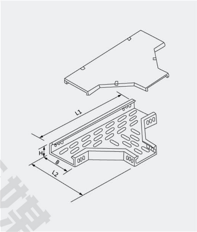
托盘式电缆桥架水平等径三通
