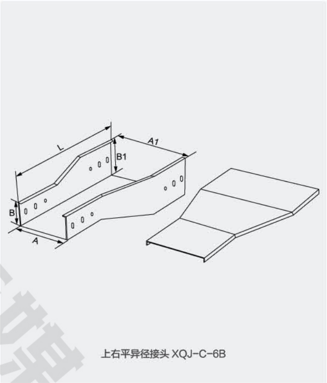
上右平异径接头
