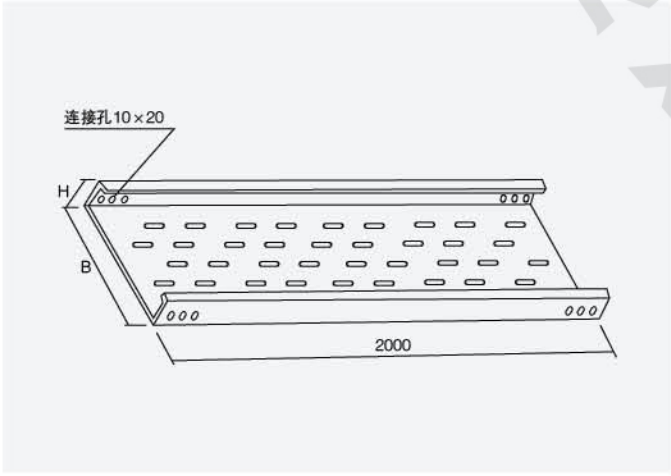
LQJ 系列铝合金电缆桥架
