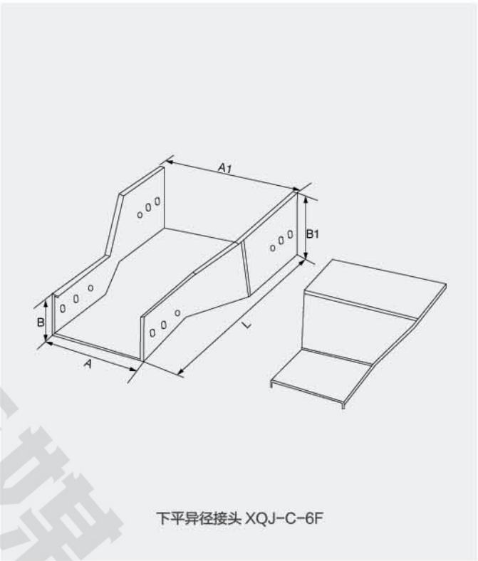
下平异径接头
